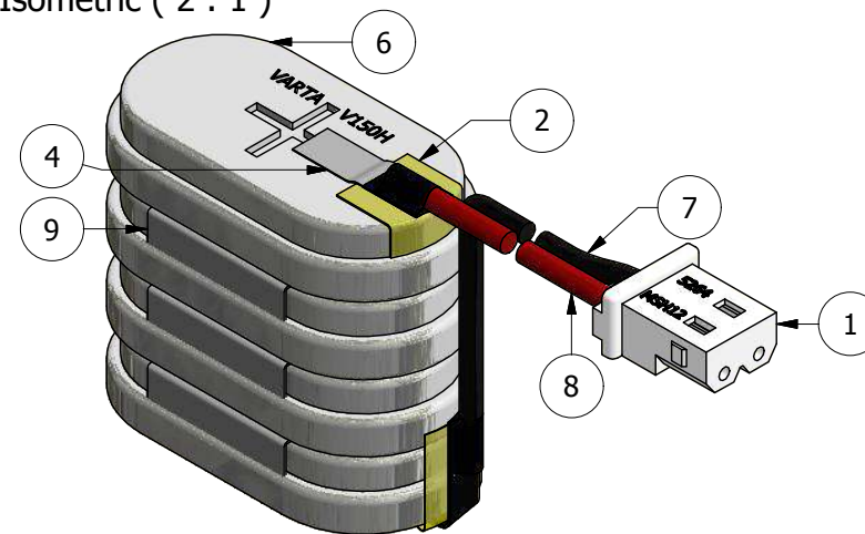
Isometric ( 2 : 1 )
